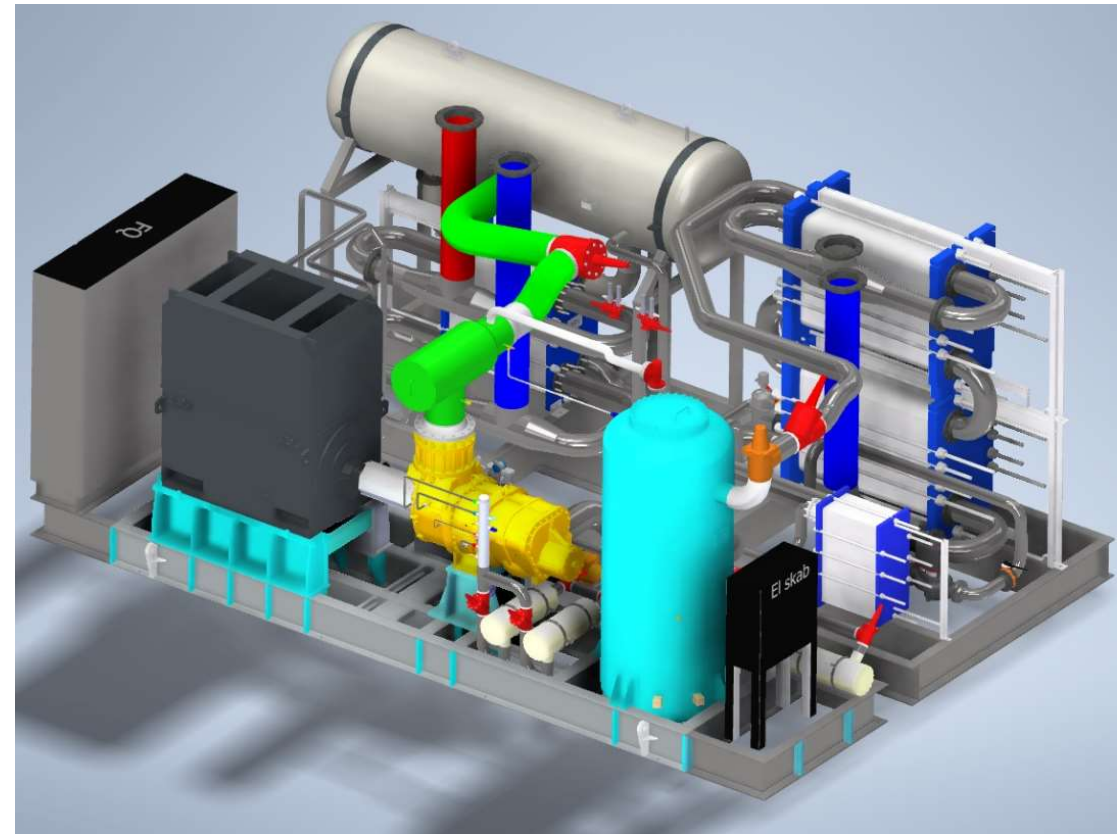
10 MW varmepumpe, Fjernvarme Fyn, afleveret Juni 2021
